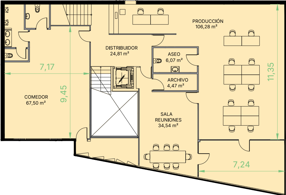
Planta Primera 331 m 2
