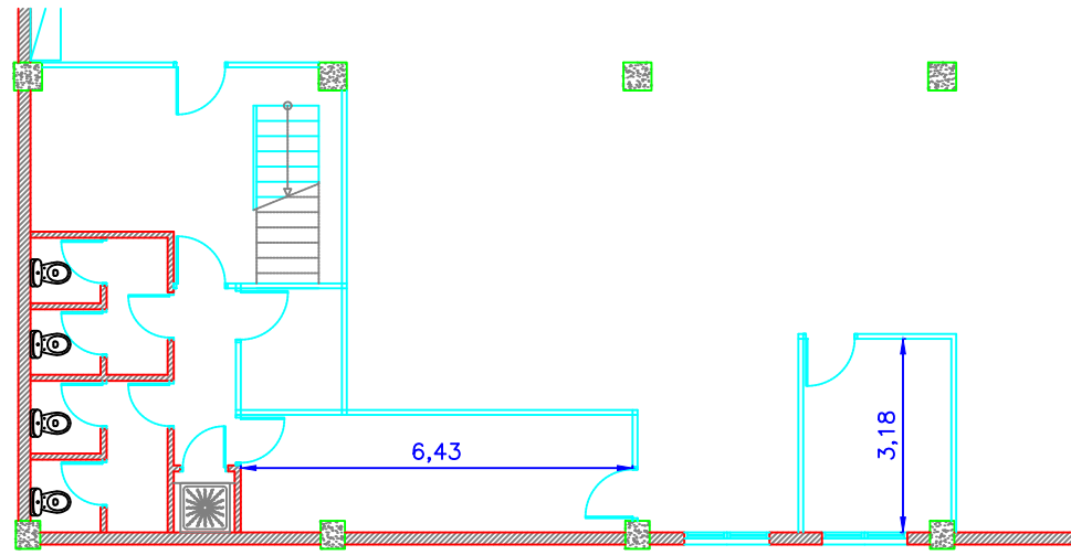
PLANTA BAJA OFICINAS
