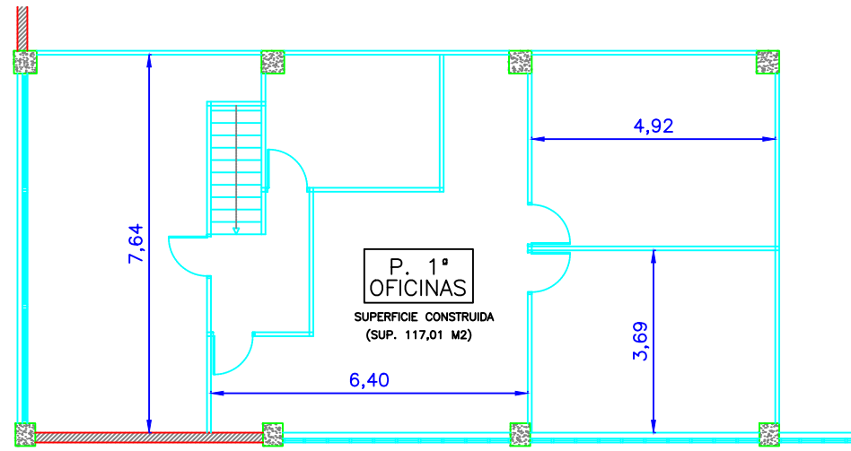
PLANTA PRIMERA OFICINAS
