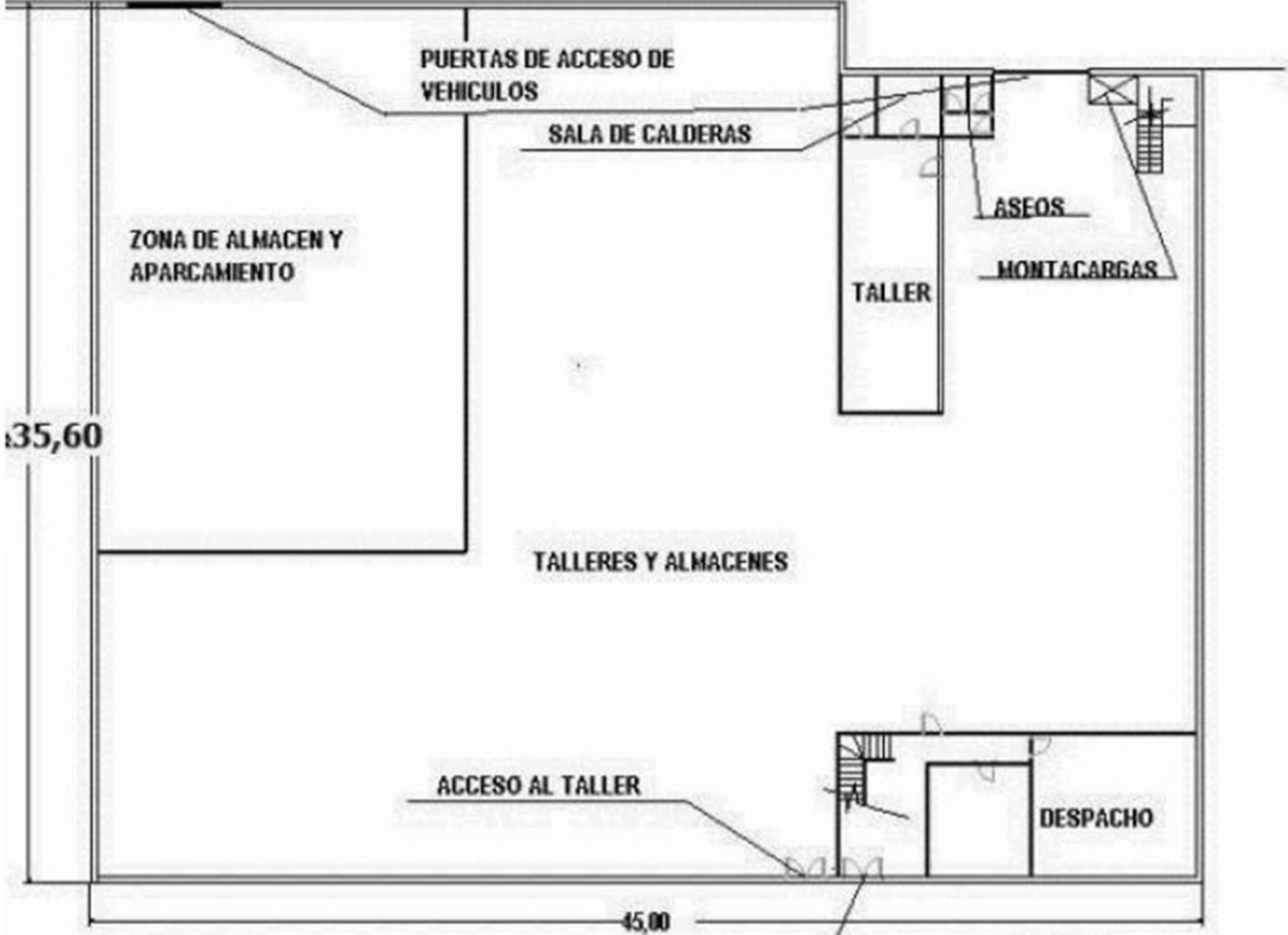
PLANTA BAJA NAVES ADOSADAS EN CEMBRANOS-LEÓN CARRETERA LEÓN-ZAMORA Km. 139
