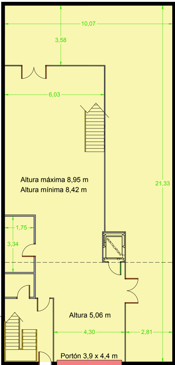
Planta baja 215 m 2 útiles
