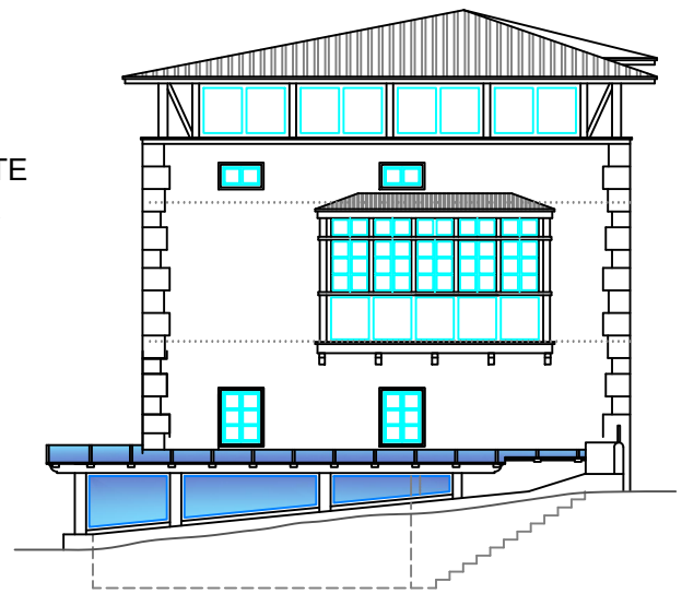
FACHADA SUR
