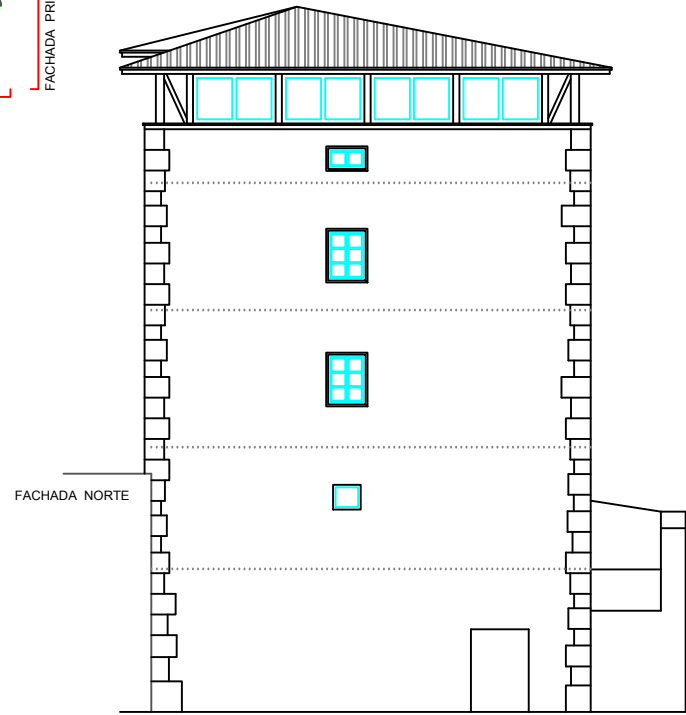
FACHADA SUR
