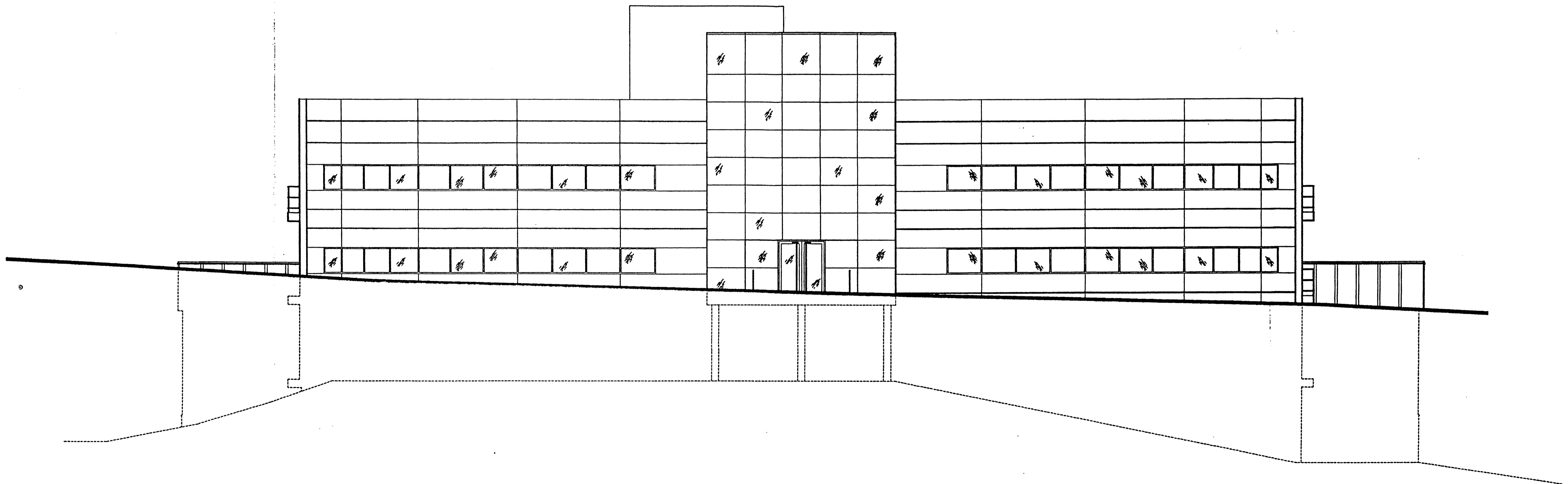
ALZADO 1 (DESDE CARRETERA).- ESCALA: 1/100.
