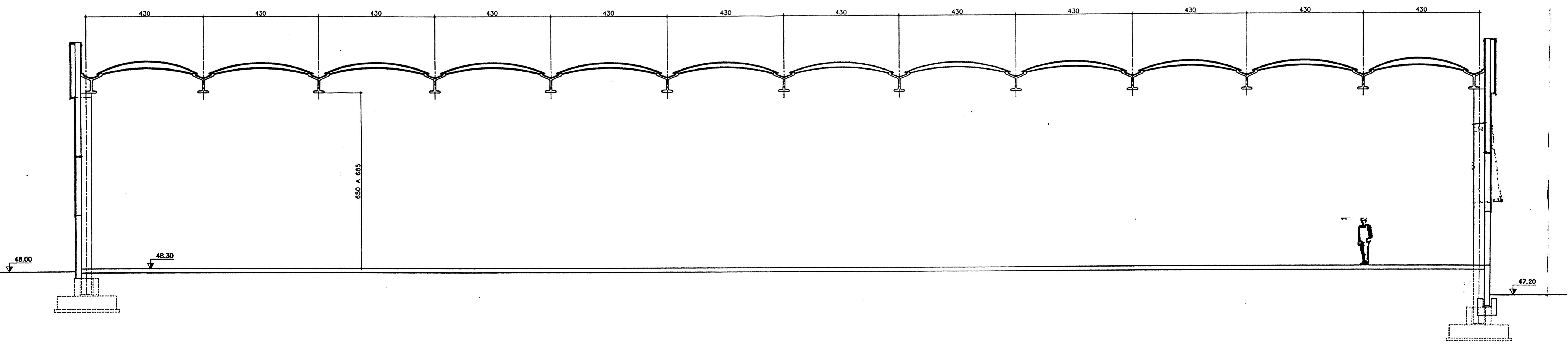
SECCION 3.- ESCALA: 1/75.
