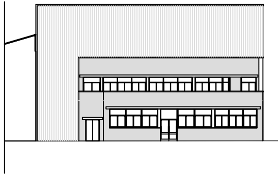
ALZADO A1
