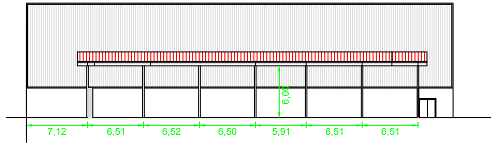
ALZADO A4
