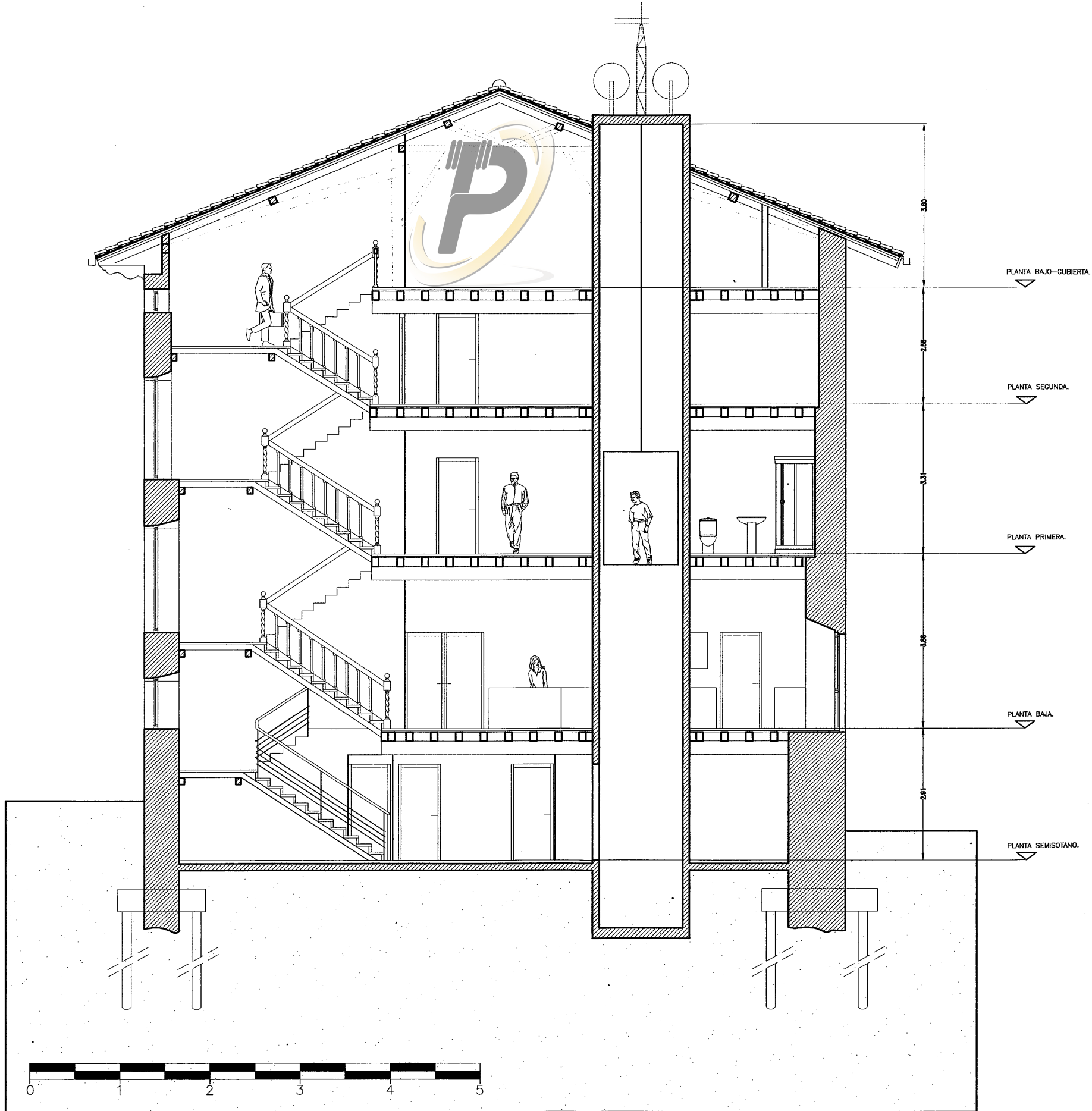
SECCION A-A'
