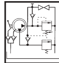
Esquema hidráulico
