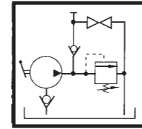
Esquema hidráulico
