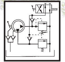
Esquema hidráulico
