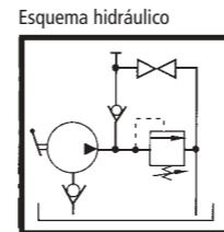
Esquema hidráulico
