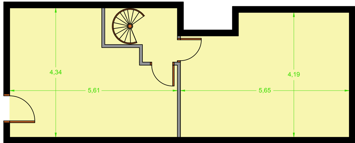
PLANTA PRIMERA - Superficie útil: 46 m 2
